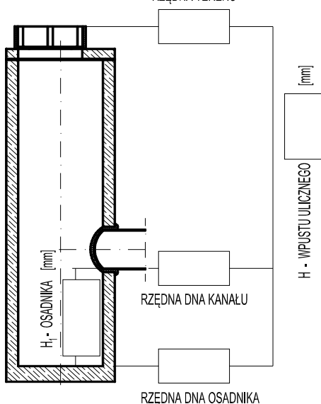
Wpust uliczny bez pierścienia odciążającego RZĘDNA TERENU
