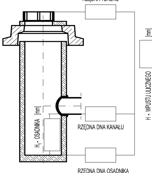
Wpust uliczny z pierścieniem odciążającym RZĘDNA TERENU
